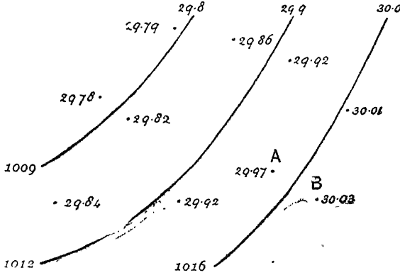
चित्र १—समदाब रेखाओं के खींचने का नियम (मिलीबार तुल्य अनुमानतः)
